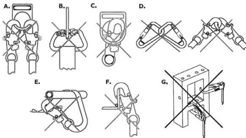
図 11 コネクタ
