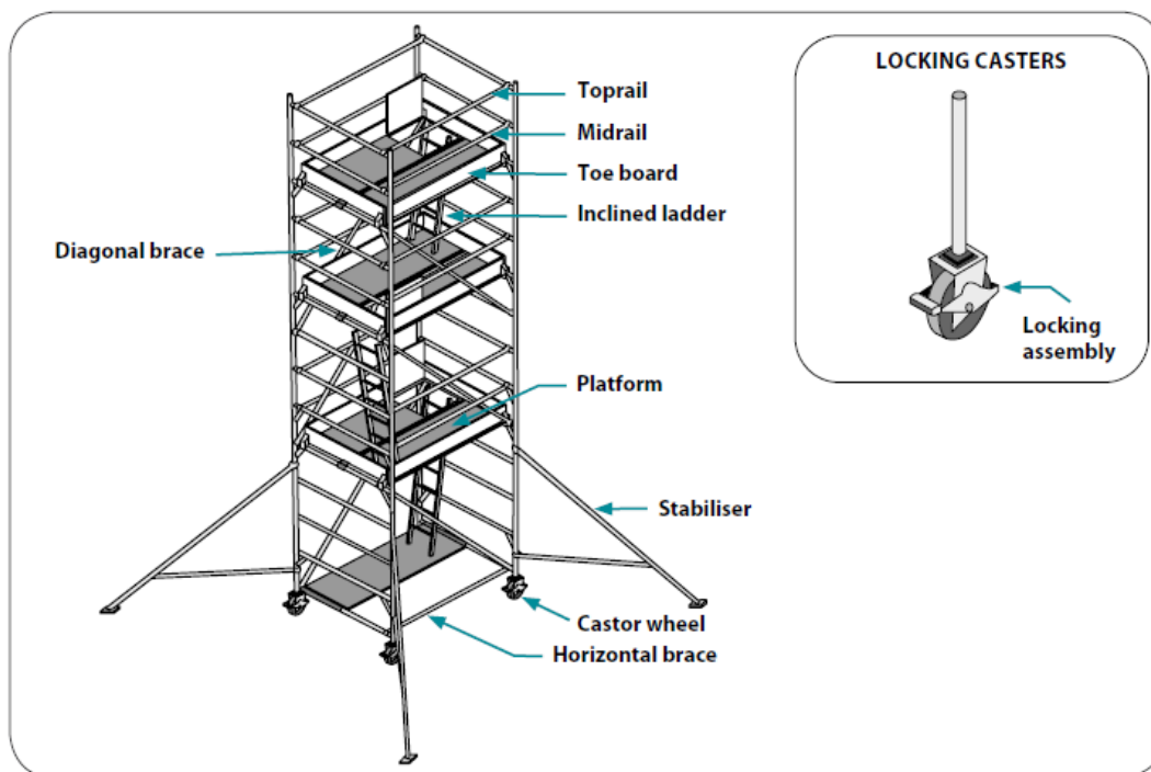
図 29 移動式塔型足場
