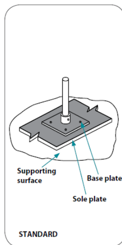
図 35 ソールプレートとベースプレート
