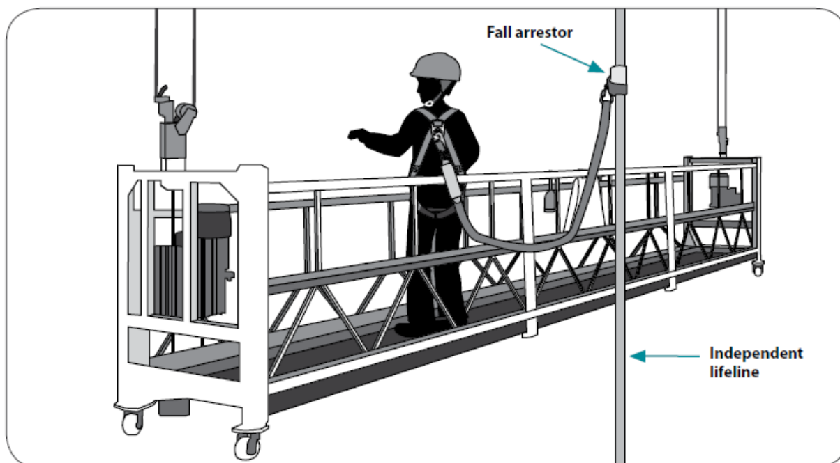
図 30 ゴンドラ
