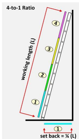
図27 伸縮式はしごの要件（4:1 の比率）
