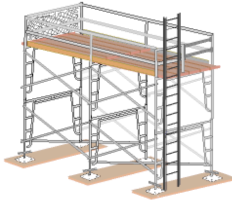
図 28 枠組み足場
