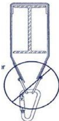
図9 タイオフアダプターの大きなDリングを通る小さなDリング
